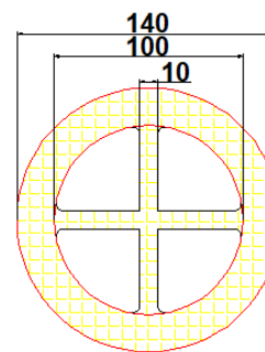
泄水孔铸铁盖俯视图
