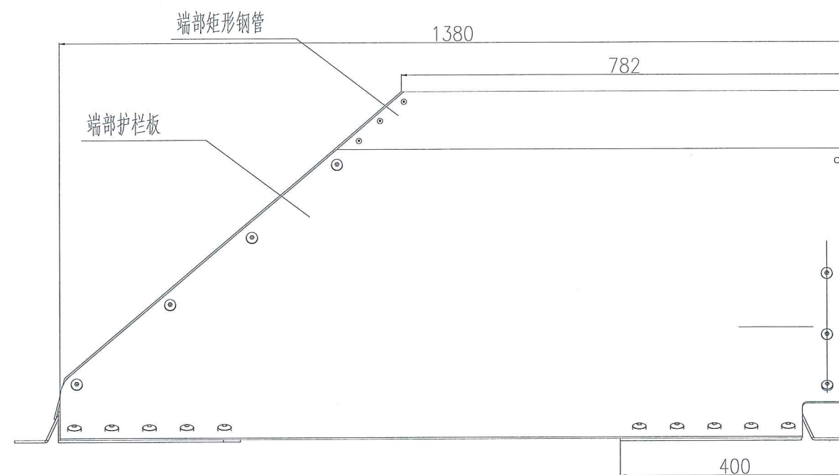
端部护栏板立面图
