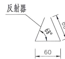
侧面图
