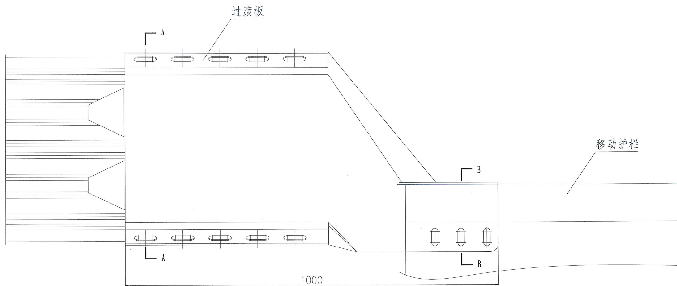
移动护栏与钢护栏连接部设计图
