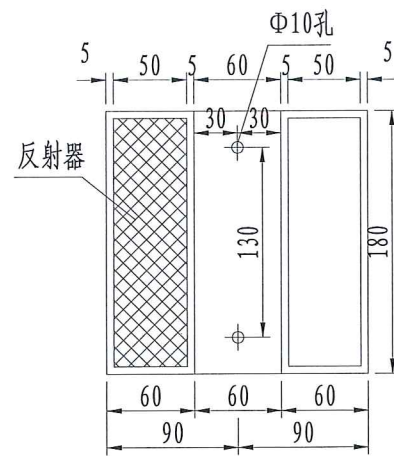
展开平面图
