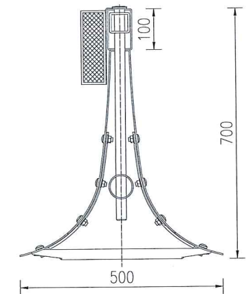
混凝土护栏轮廓安装立面图
