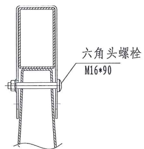
B-B 1:1
