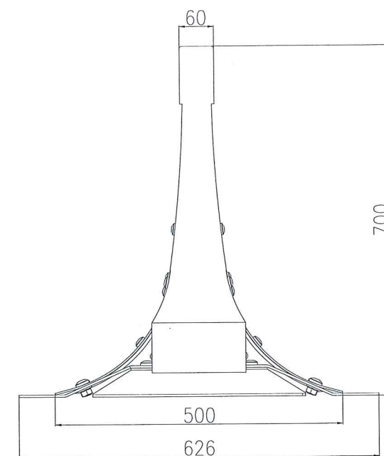
端部护栏板剖面图
