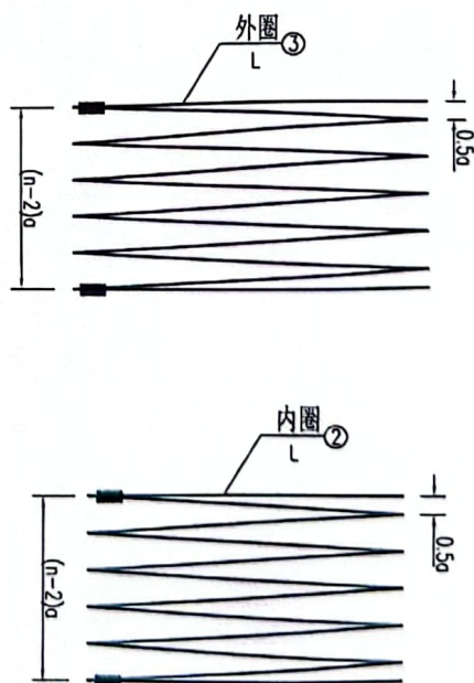
螺旋钢筋示意
