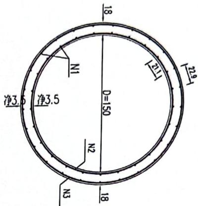
横断面
