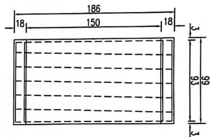
纵断面
